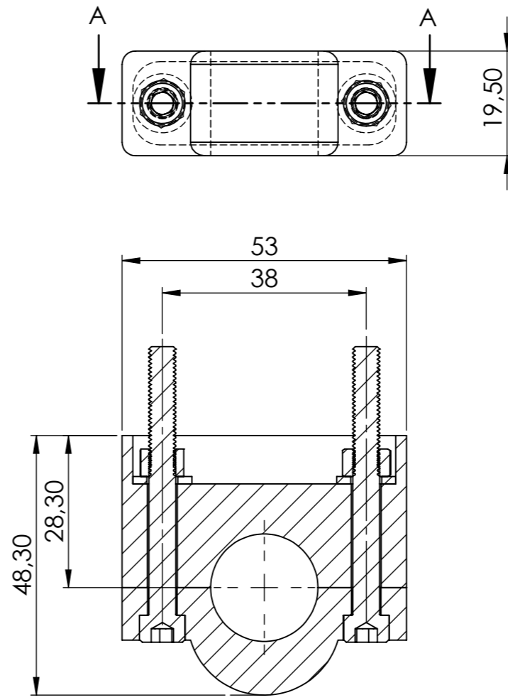
SEÇÃO A-A
