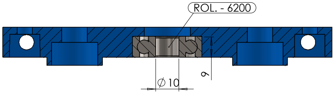
SEÇÃO A-A
