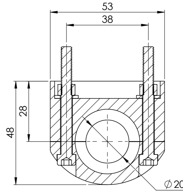
SEÇÃO A-A
